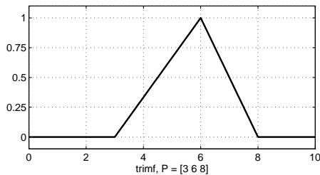
trimf
